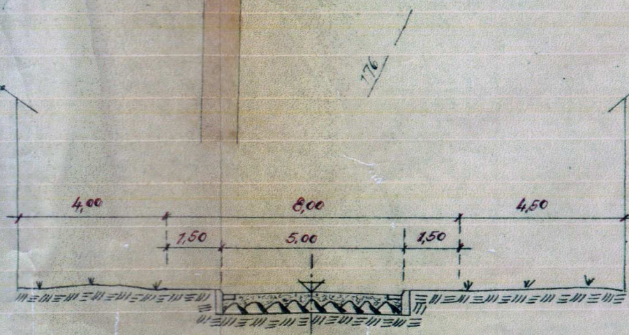
STRASSENPROFIL 1:100
