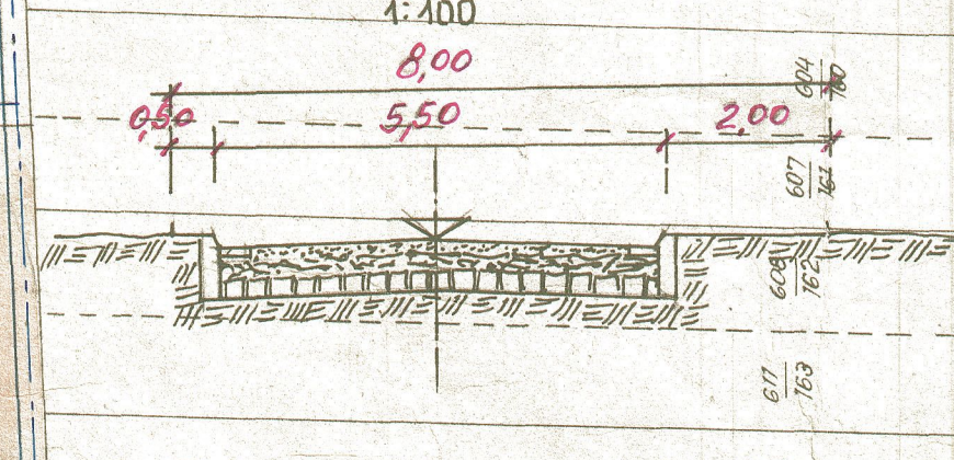
STRASSENPROFIL "B"
