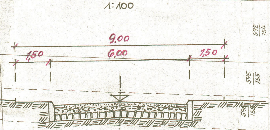
STRASSENPROFIL "A"
