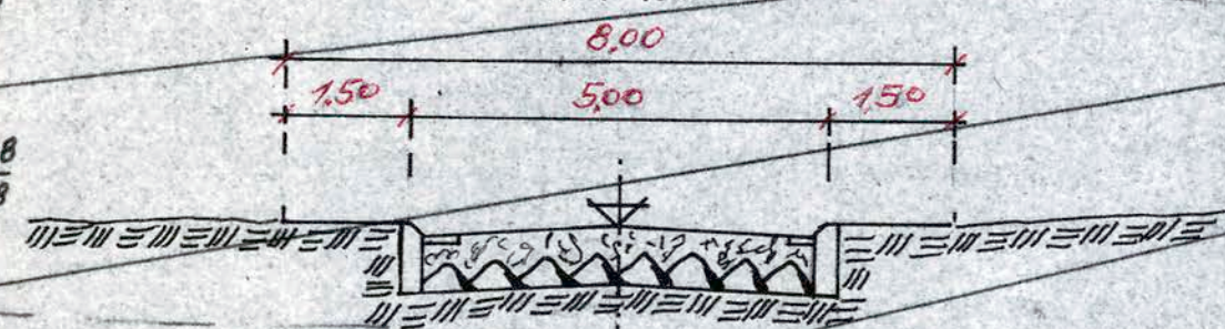
STRASSENPROFIL „A“ M. 1:100
