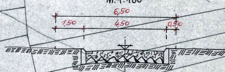
STRASSENPROFIL „B“ M. 1:100
