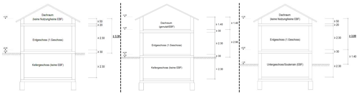
Abbildung 3: Festlegung der Geschosshöhen zur Ermittlung der Stockwerksanzahl 5
